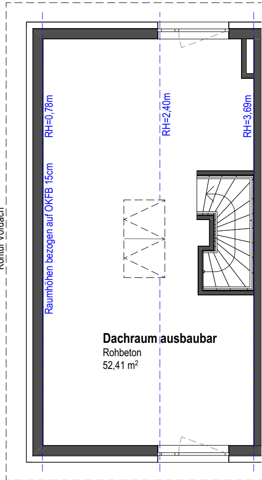
5A - Dachgeschoss
