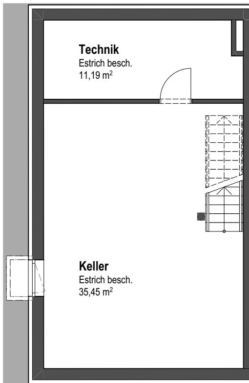
8A - Untergeschoss
