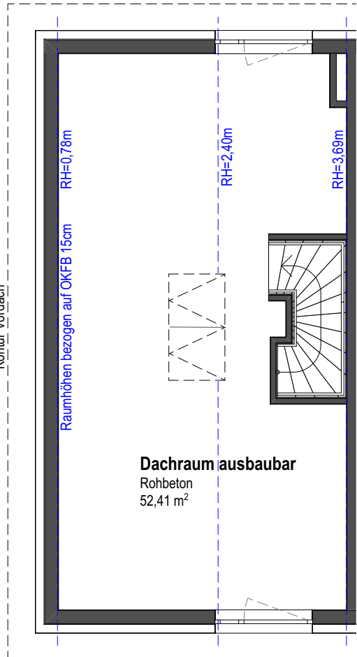
6A - Dachgeschoss
