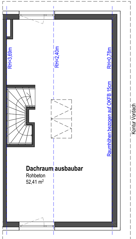
5B - Dachgeschoss
