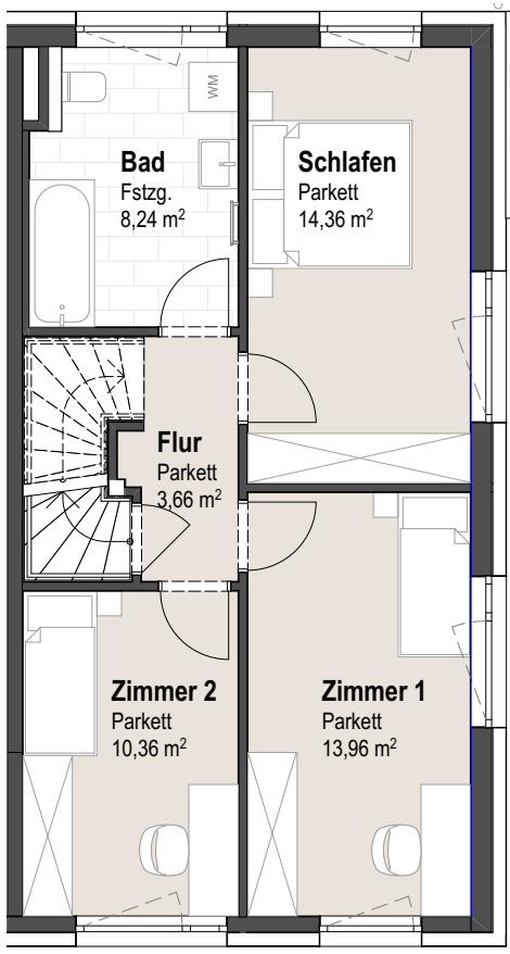
5B - Obergeschoss
