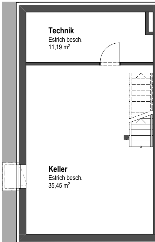
8B - Untergeschoss
