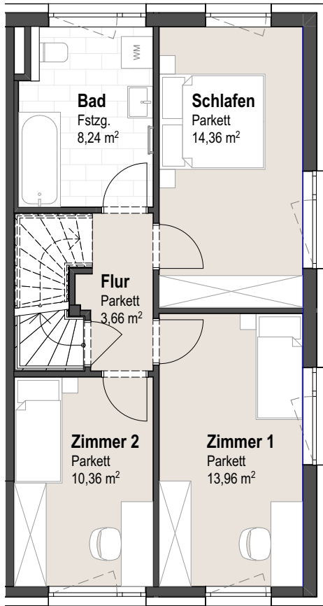
7B - Obergeschoss
