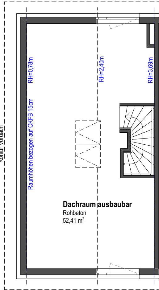
8A - Dachgeschoss
