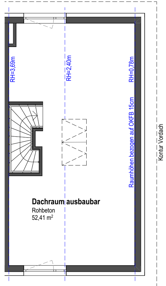
8B - Dachgeschoss
