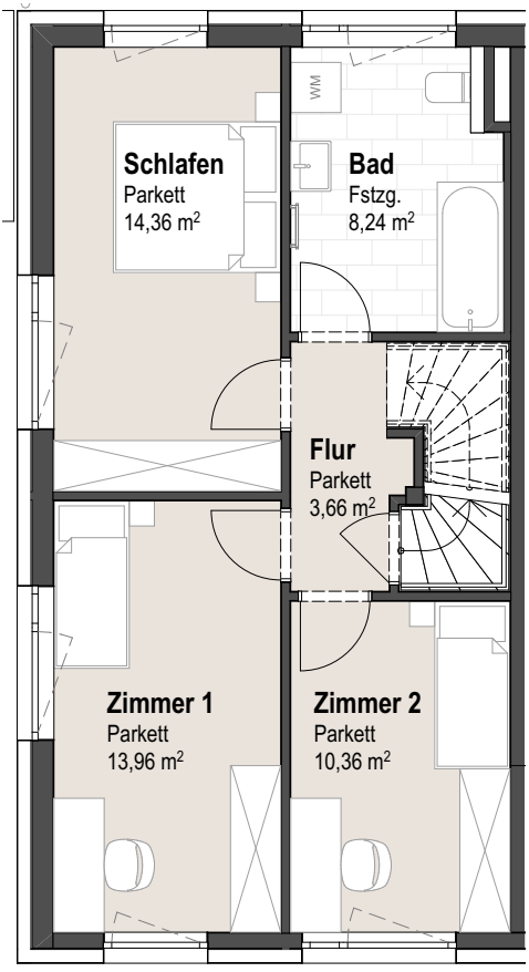
7A - Obergeschoss
