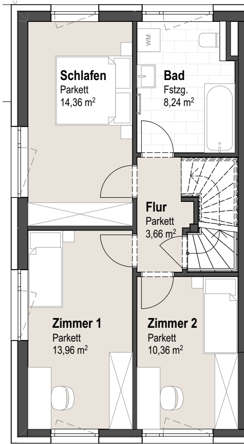
8A - Obergeschoss
