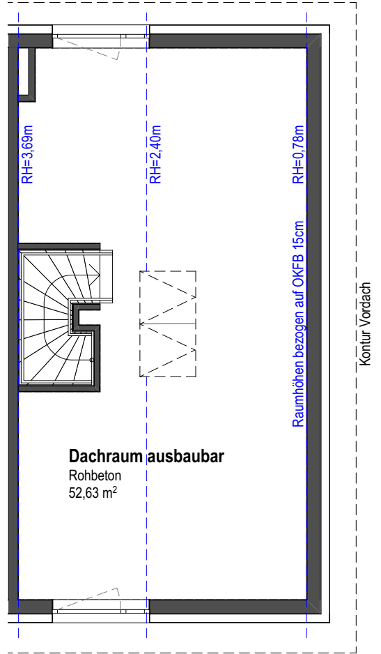
2A - Dachgeschoss
