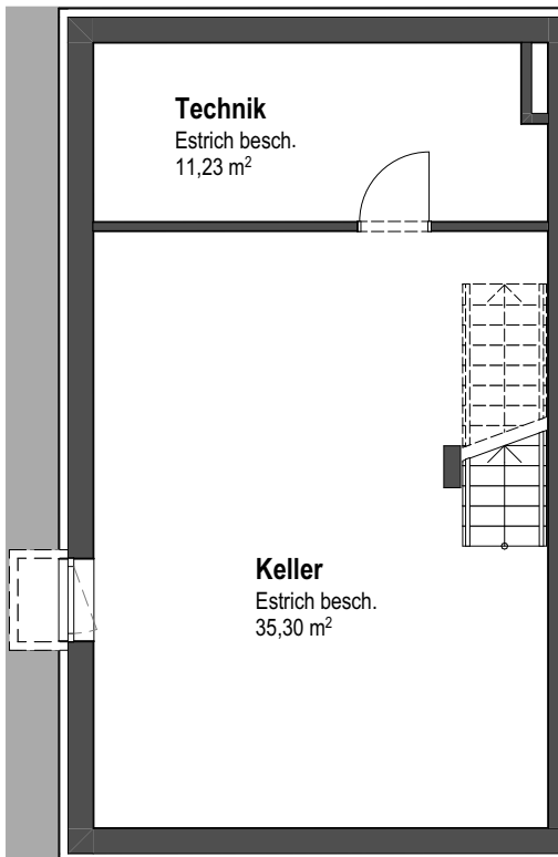
1B - Untergeschoss
