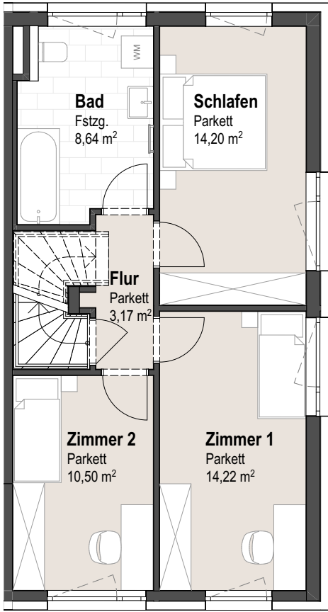
2A - Obergeschoss
