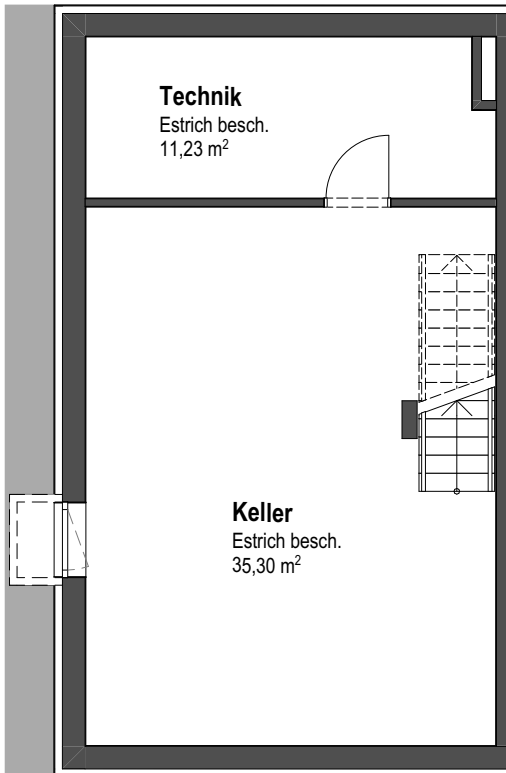
2B - Untergeschoss
