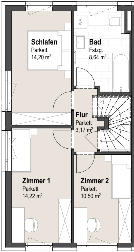
2B - Obergeschoss
