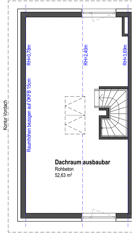
2B - Dachgeschoss
