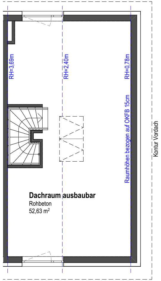
4A - Dachgeschoss Datum: 2023-06-23 Gez.: PE
