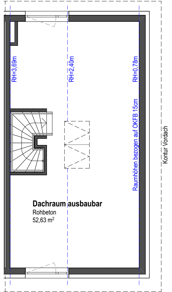
3A - Dachgeschoss
