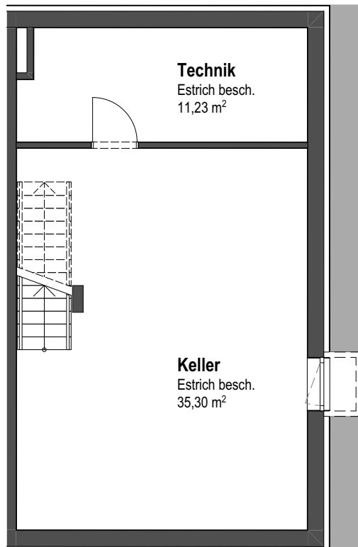
3A - Untergeschoss
