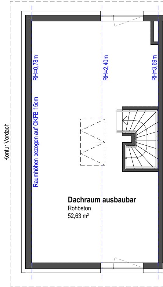
4B - Dachgeschoss
