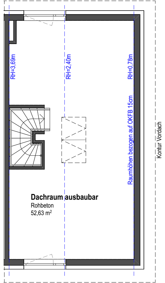
1A - Dachgeschoss
